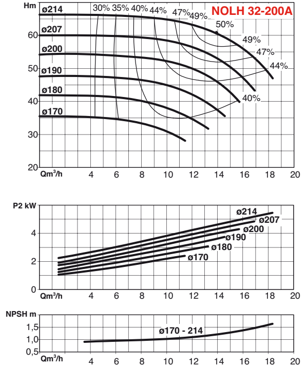
Facteur Q min./Q nom. 0,3 Facteur Q max./Q nom. 1,2 NOLH 32-200A
