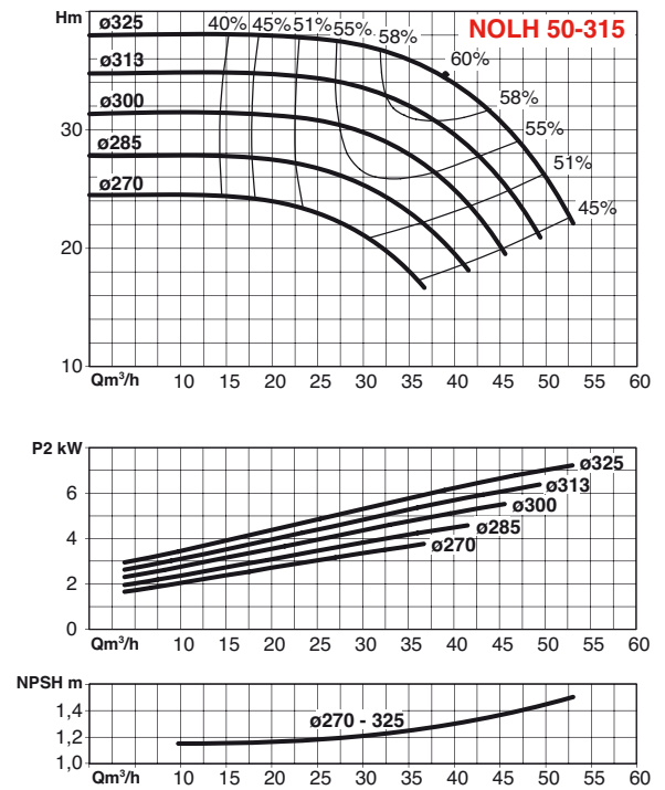
Facteur Q min./Q nom. 0,3 Facteur Q max./Q nom. 1,2 NOLH 50-315
