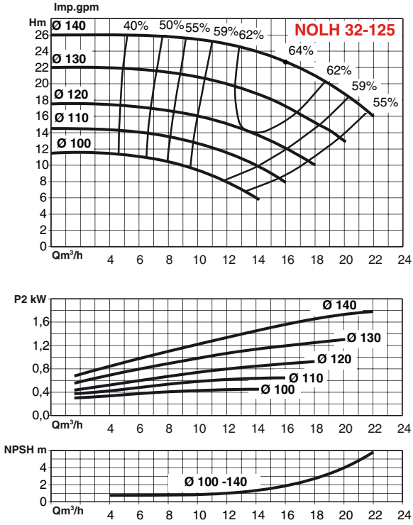
Facteur Q min./Q nom. 0,3 Facteur Q max./Q nom. 1,2 NOLH 32-125
