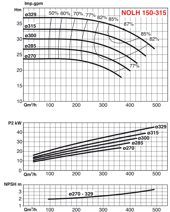
Facteur Q min./Q nom. Facteur Q max./Q nom. NOLH 150-315 0,3 1,2
