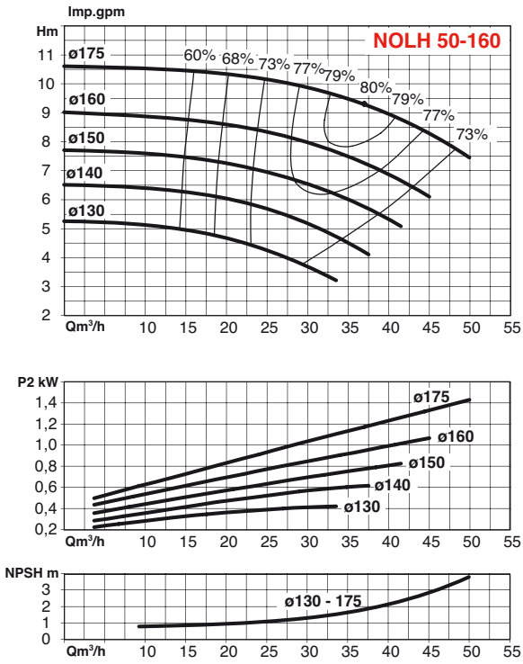
Facteur Q min./Q nom. 0,3 Facteur Q max./Q nom. 1,2 NOLH 50-160
