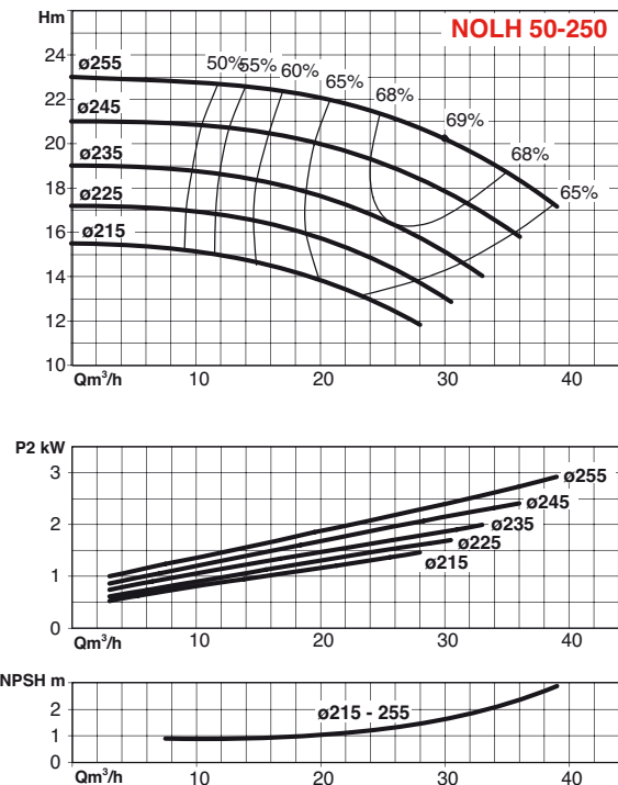
Facteur Q min./Q nom. 0,3 Facteur Q max./Q nom. 1,2 NOLH 50-250
