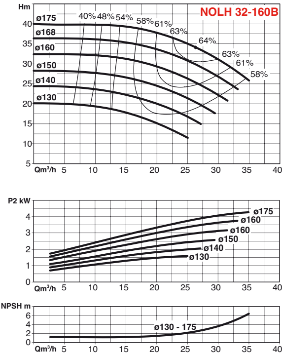
Facteur Q min./Q nom. 0,3 Facteur Q max./Q nom. 1,2 NOLH 32-160B
