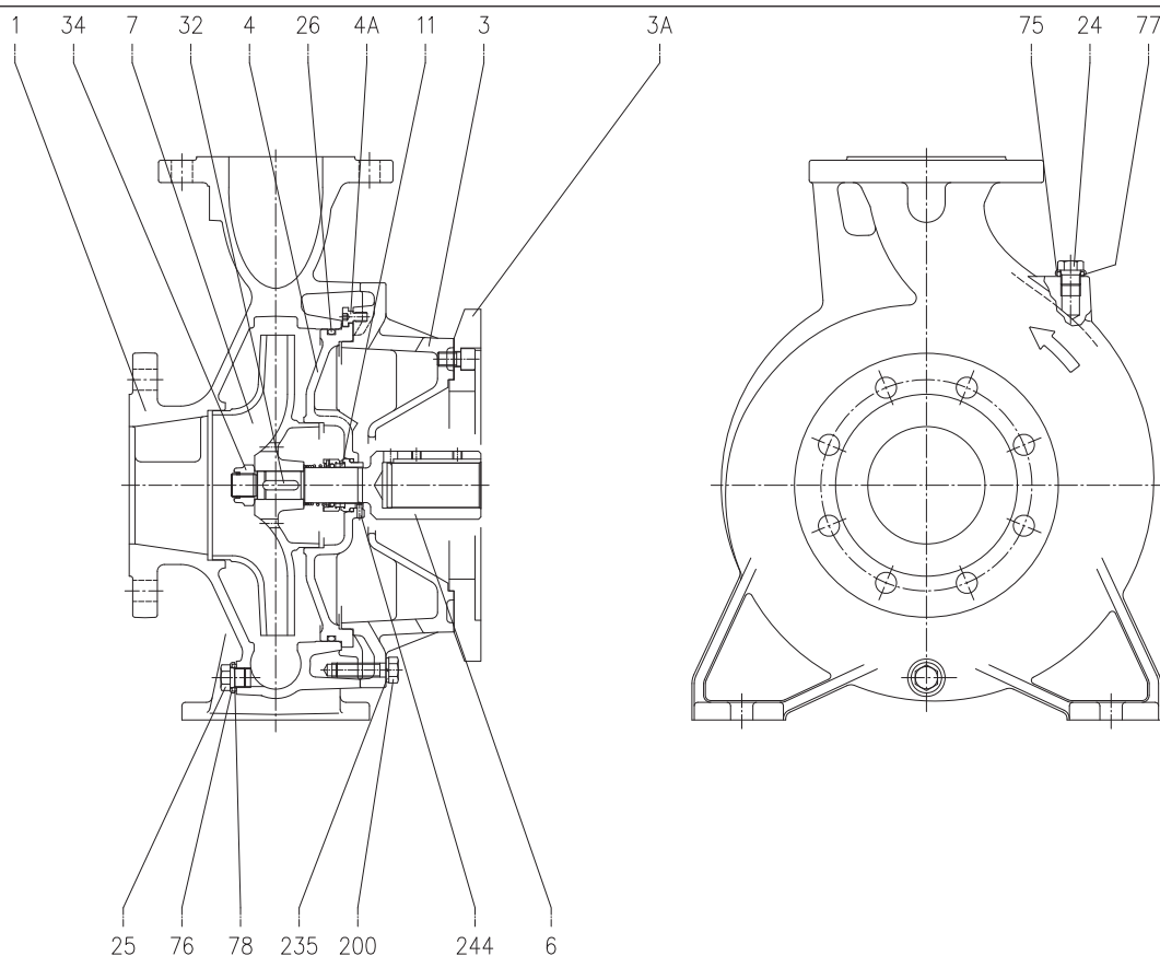
VUE EN COUPE SÉRIE 3LSF4 65-250, 80
