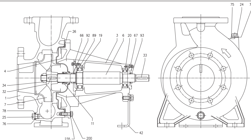
VUE EN COUPE SÉRIE 3LP4 80-160
