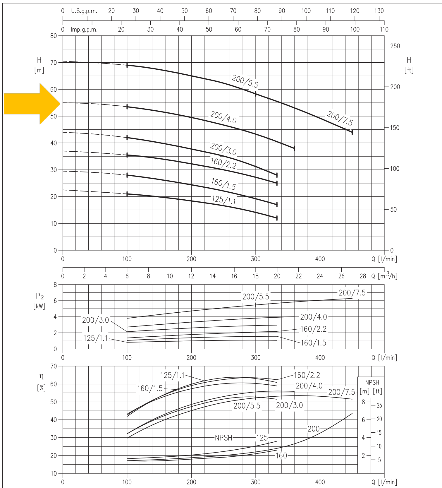
COURBES DE PERFORMANCE SÉRIE 3(L)M-3(L)S-3(L)P 32 à 2900 min -1 (selon ISO 9906 Annexe A)
